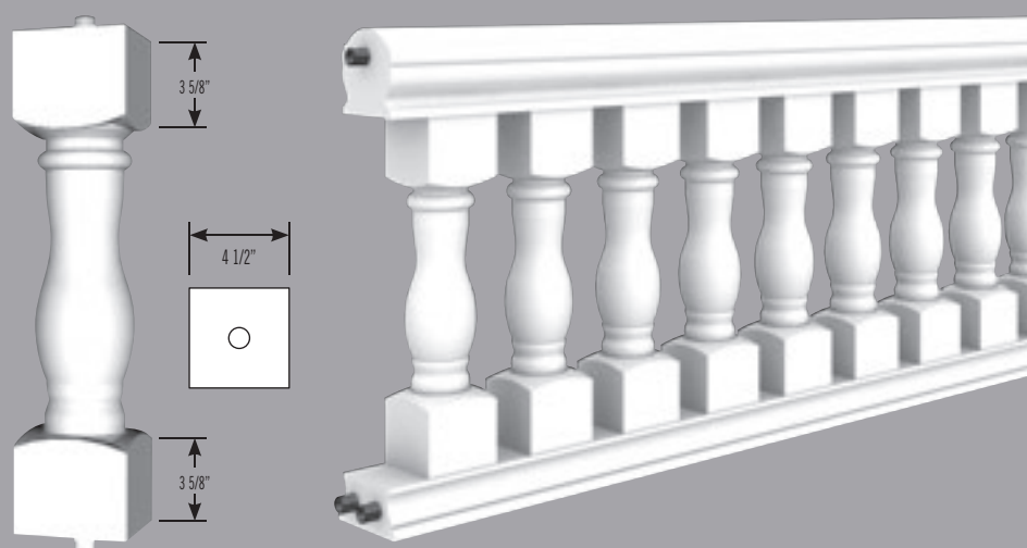
1324 Balustre Baluster
