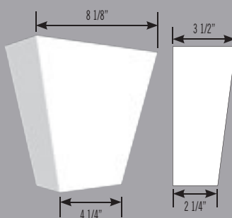
7057 Clé de voûte Keystone L/W: 8 1/8" H: 7 3/4" P: 3 1/2"
