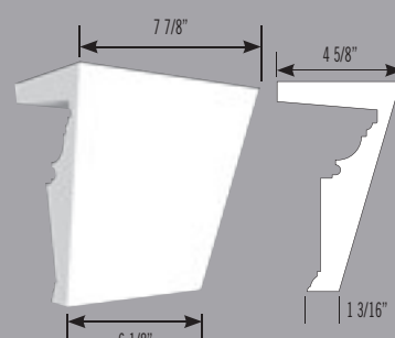
7055-1 Clé de voûte profilée Shaped Keystone L/W: 7 7/8" H: 7 7/8" P: 4 5/8"
