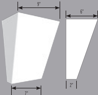
7056 Clé de voûte Keystone
