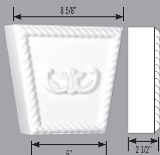
5508 Clé de voûte Keystone L/W: 8 5/8" H: 7 1/2" P: 2 1/2"
