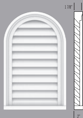
9814-22 L/W: 14" H: 22" P: 2" 9814-36 L/W: 14" H: 36" P: 2" 9814-S L/W: 14" H: 14 à/to 35" P: 2"
