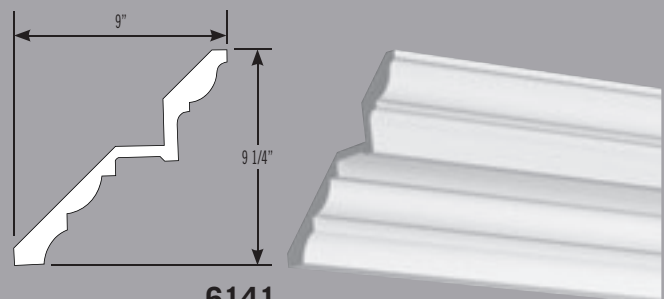
6141 Moulure à corniche Cornice Moulding H: 9 1/4" P: 9" Lg: 192"
