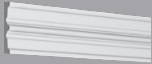
6004 Moulure de portes et fenêtres Door and Window Moulding H: 4" P: 5/8" Lg: 96"
