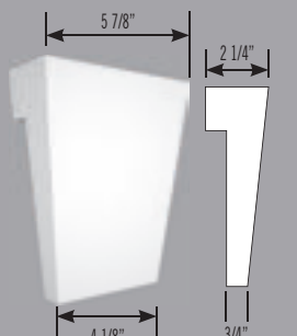
7054 Clé de voûte Keystone L/W: 5 7/8" H: 7 1/8" P: 2 1/4"
