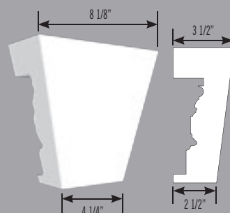
7072 Clé de voûte profilée Shaped Keystone L: 8 1/8" H: 7 3/4" P: 3 1/2"
