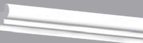
6007-N2 Moulure-cadre Frame Moulding H: 1 11/16" P: 1 3/16" Lg: 192"
