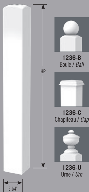
1236 Poteau de rampe Newel Post
