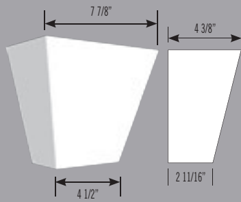
7022 Clé de voûte Keystone
