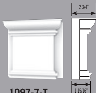
1097-7-T Tête de pilastre Pilaster Head L/W: 7" H: 6 7/8" P: 2 3/4"
