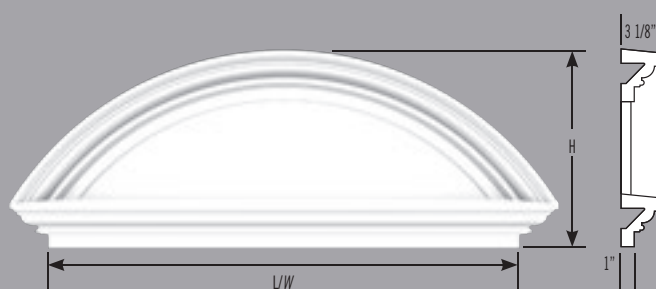
Fronton en segment Segment Pediment
