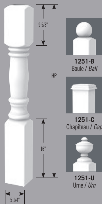
1251 Poteau de rampe Newel Post
