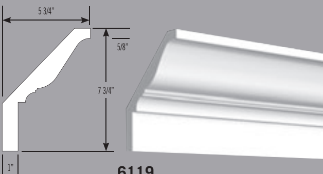
6119 Moulure à fascia et couronne Crown Fascia Moulding H: 7 3/4" P: 5 3/4" Lg: 192"
