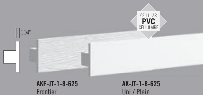
AK-JT & AKF-JT Cache-joint uni en T pour planches et soffites T-Shaped Plain Joint Cover for Boards and Soffits L/W: 1 1/4" P: 5/8" Lg: 96"
