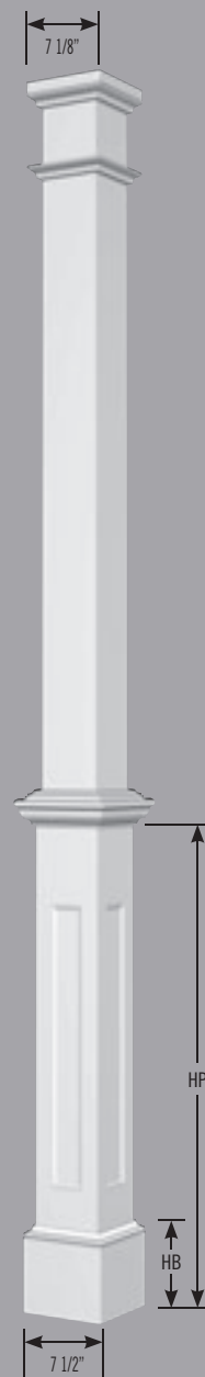
1202 Colonne à fût carrée Square Column
