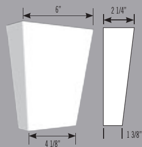
7006 Clé de voûte Keystone L/W: 6" H: 7 1/8" P: 2 1/4"
