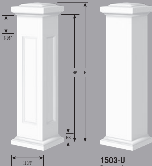
1503 Poteau de rampe Newel Post
