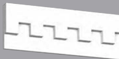
6121 Moulure à fascia dentelée Dentil Fascia Moulding H: 7 3/16" P: 1 5/8" Lg: 192" Rep: 4"
