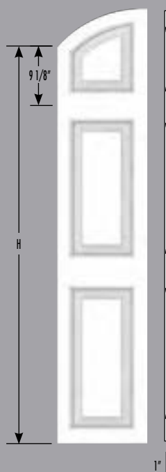
6514-2-QS9-I Volet à deux panneaux soulevés identiques avec tête 6514-QS9 Raised Two Identical Panel Shutter with 6514-QS9 Head
