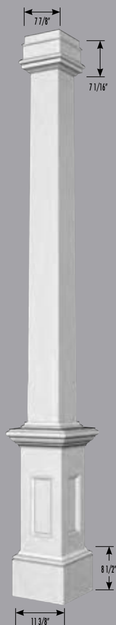
1500-F-09 Colonne à fût carré en fuseau Tapered Square Column
