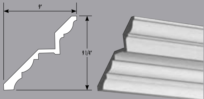
6141 Moulure à corniche Cornice Moulding H: 9 1/4" P: 9" Lg: 192"
