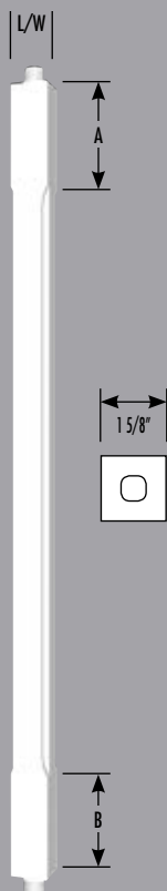
1228 Balustre Baluster
