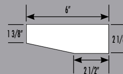
6118-SO Socle pour 6118 Base Block for 6118 L/W: 6" H: 9" P: 2 1/8"
