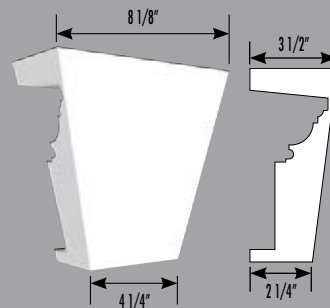
7057-1 Clé de voûte profilée Shaped Keystone L/W: 8 1/8" H: 7 3/4" P: 3 1/2"
