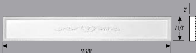
5507 Tête décorative Decorative Crosshead L/W: 55 5/8" H: 7 1/2" P: 2"
