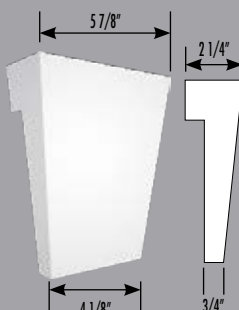
7054 Clé de voûte Keystone L/W: 5 7/8" H: 7 1/8" P: 2 1/4"
