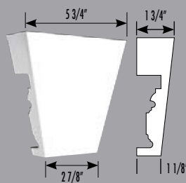
7005-1 Clé de voûte profilée Shaped Keystone L/W: 5 3/4" H: 5 1/2" P: 1 3/4"
