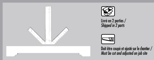
4371 Ornement de pignon Gable Ornament L/W: 72" H: 42" P: 1" Pente/Pitch: 8/12 à/to 14/12
