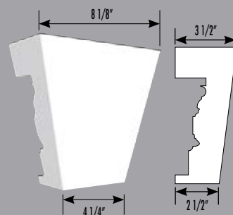
7072 Clé de voûte profilée Shaped Keystone L/W: 8 1/8" H: 7 3/4" P: 3 1/2"
