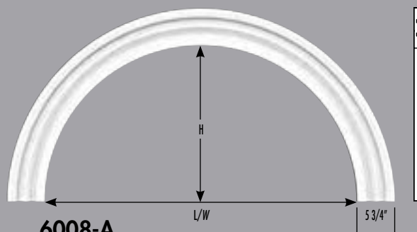
6008-A Arche en demi-cercle Half Circle Arch L/W: sur mesure/custom sized H: sur mesure/custom sized P: 1 1/8"
