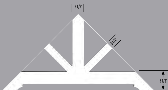
4371 Ornement de pignon Gable Ornament L/W: 72" H: 42" P: 1" Pente/Pitch: 8/12 à/to 14/12
