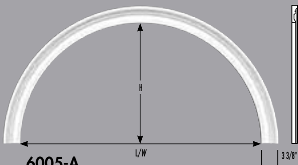
6005-A Arche en demi-cercle Half Circle Arch L/W: sur mesure/custom sized H: sur mesure/custom sized P: 1 1/8"
