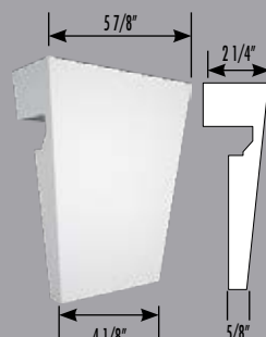
7054-1 Clé de voûte profilée Shaped Keystone L/W: 5 7/8" H: 7 1/8" P: 2 1/4"
