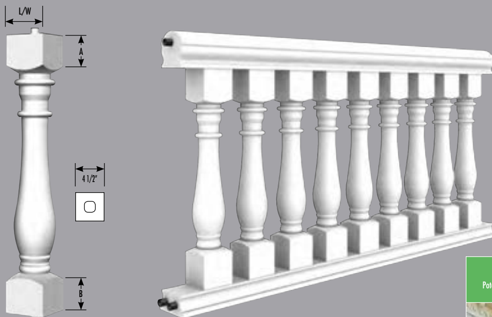
1320 Balustre Baluster
