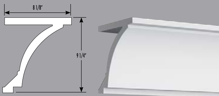
6164 Moulure en baie Cove Moulding H: 9 1/4" P: 8 1/8" Lg: 192"
