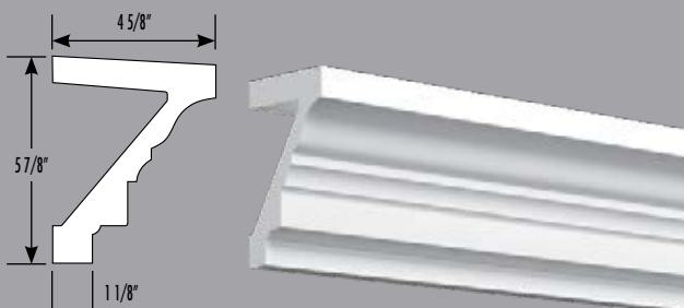
6156-B NOUVEAU NEW Moulure de corniche Cornice Moulding H: 5 7/8" P: 4 5/8" Lg: 131"
