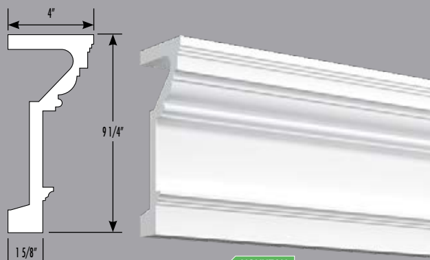
6186 NOUVEAU NEW Moulure de corniche Cornice Moulding H: 9 1/4" P: 4" Lg: 143"
